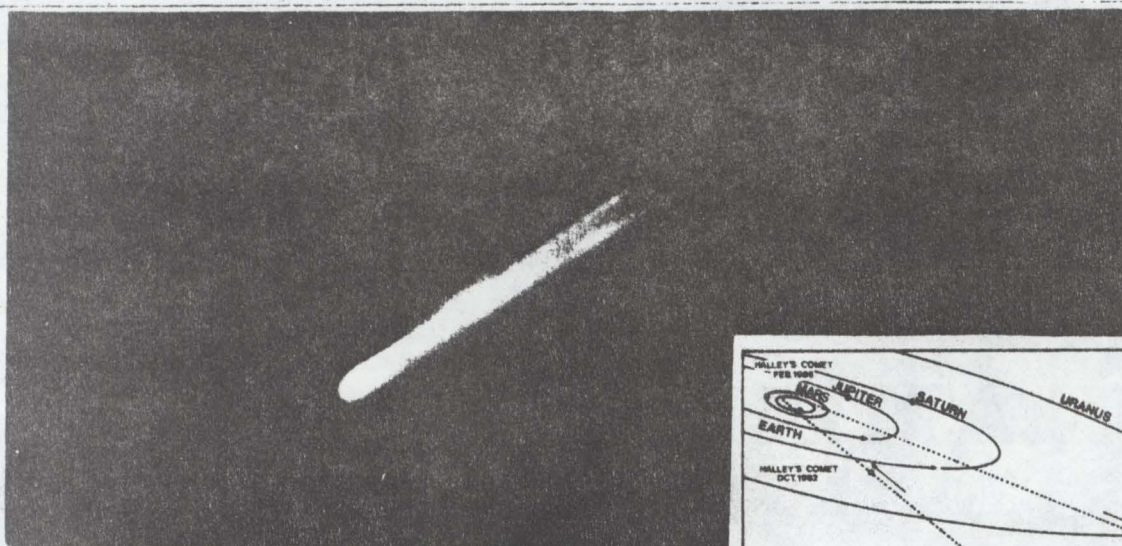
Bild. Halleys Komet och dess bana runt solen.
